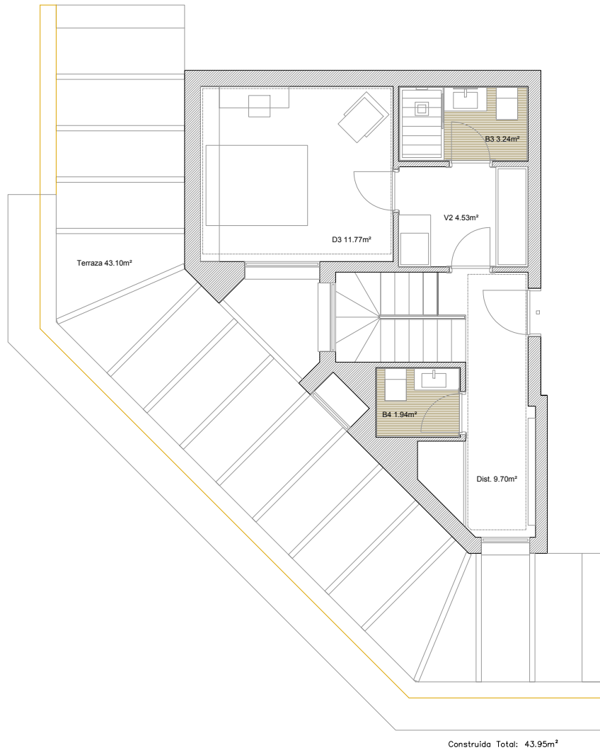
ALTERNATIVA VIVIENDA BAJO CUBIERTA
